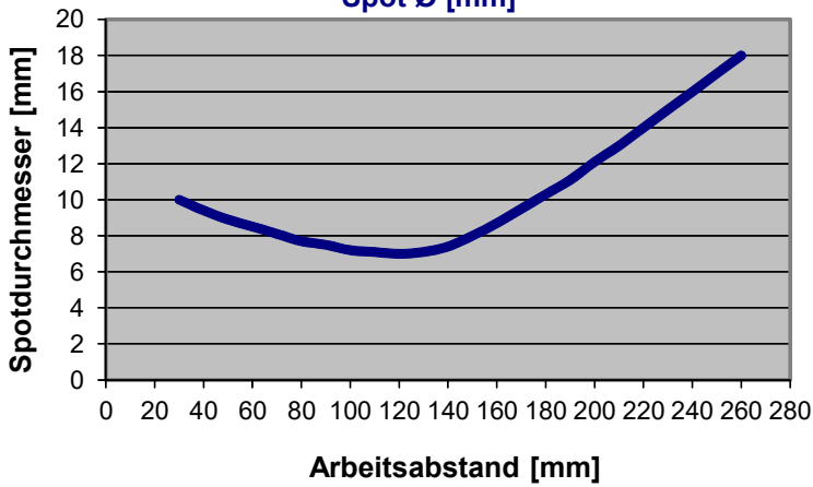
KL-M34-XL-A2.0 (fokussiert auf 140 mm) + R-S-A2.0-(2.5)-1200-67° Spot Ø [mm]
