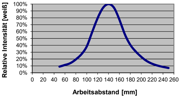
KL-M34-XL-A1.1 (fokussiert auf 140 mm) + R-S-A1.1-(1.5)-1200-67° INT [relativ]
