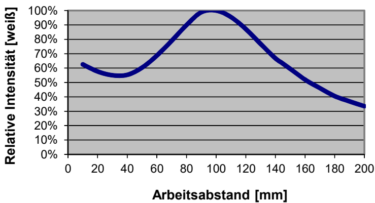
KL-M18-XL-A2.0 (fokussiert auf 140 mm) + R-S-A2.0-(2.5)-1200-67° INT [relativ]
