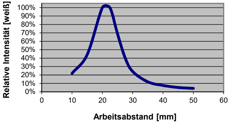
KL-M12-XL-A2.0 (fokussiert auf 25 mm) + R-S-A2.0-(2.5)-1200-67° INT [relativ]
