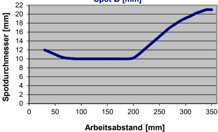
KL-M34-XL-A2.0 (fokussiert auf 240 mm) + R-S-A2.0-(2.5)-1200-67° Spot Ø [mm]
