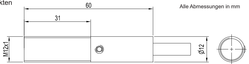
KL-M12-A2.0 mit R-S-A2.0-(2.5)-600-67°: (fokussiert auf Abstand 35 mm):
