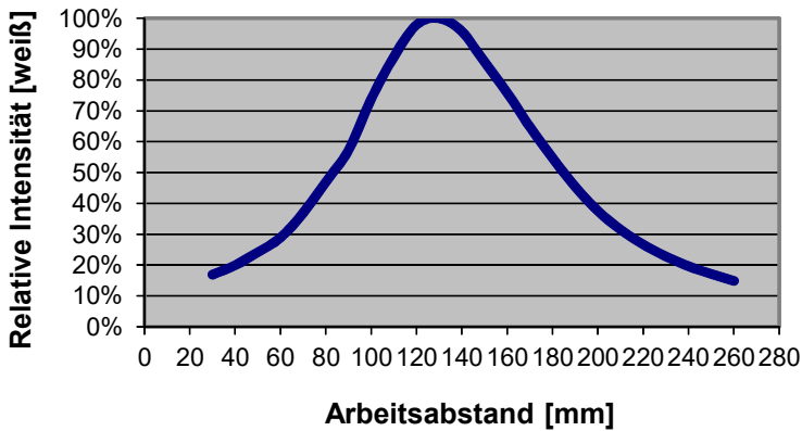
KL-M34-XL-A2.0 (fokussiert auf 140 mm) + R-S-A2.0-(2.5)-1200-67° INT [relativ]
