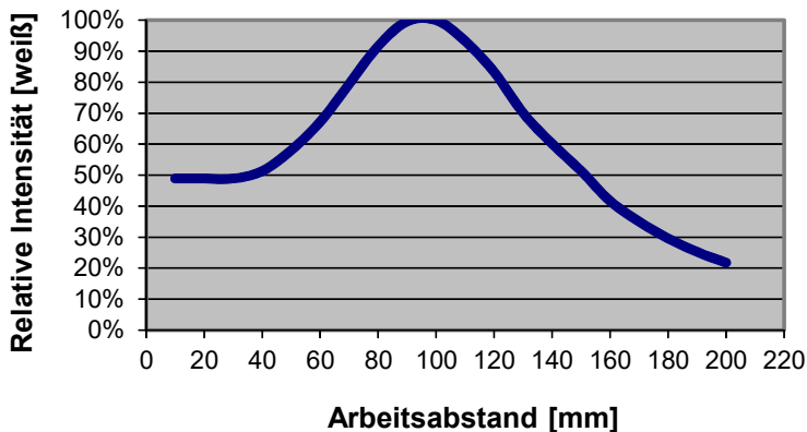
KL-M18-XL-A2.0 (fokussiert auf 200 mm) + R-S-A2.0-(2.5)-1200-67° INT [relativ]
