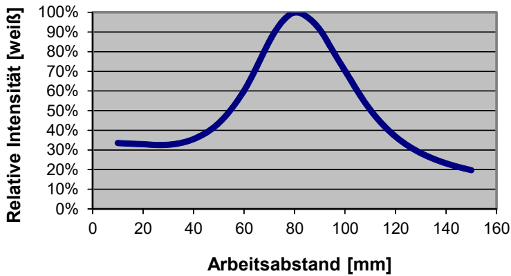
KL-M18-XL-A2.0 (fokussiert auf 80 mm) + R-S-A2.0-(2.5)-1200-67° INT [relativ]
